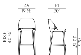
942/AW sgabello alto \ barstool
