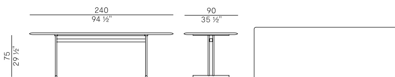
955/TR tavolo \ table
