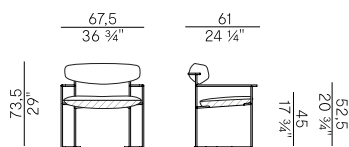
922/LMB-OUT poltrona lounge \ lounge armchair
