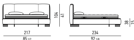
LETTO KING SIZE CM 217X234 H104 BED KING SIZE CM 217X234 H104
