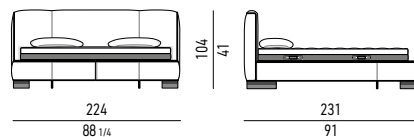
LETTO CM 224X231 H104 BED CM 224X231 H104
