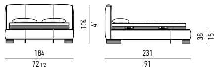
LETTO CM 184X231 H104 BED CM 184X231 H104
